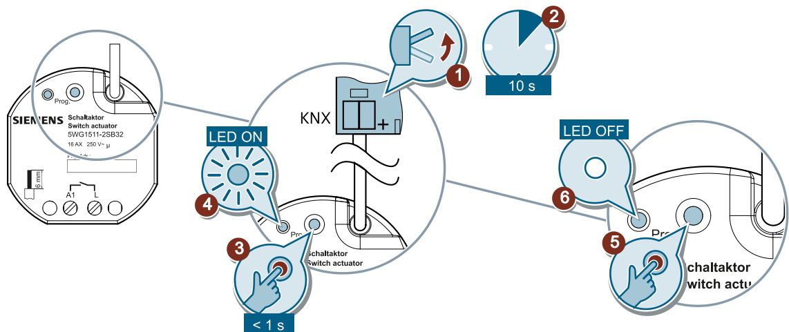
Fig. 4: Test KNX 24 V DC type SELV
