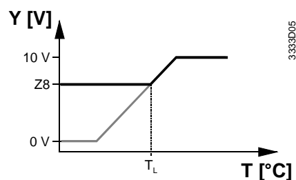
1-stopniowe chłodzenie Maksymalne ograniczenie regulowanej temperatury przez ograniczenie minimum wyjścia chłodzenia
