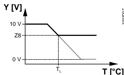
1-stopniowe ogrzewanie Minimalne ograniczenie regulowanej temperatury
