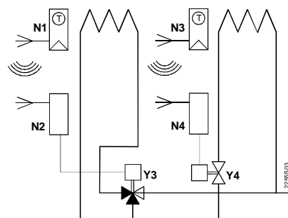
Zawór strefowy
