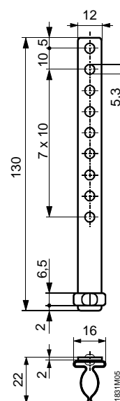
Listwa aluminiowa ARG22.2
