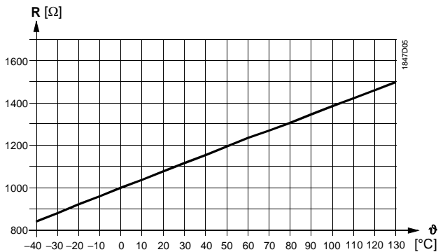
Pt 1000 (klasa B)
